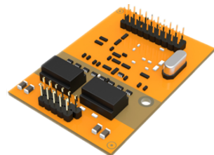
Модуль B2 2 порта BRI
